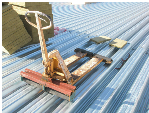
Pallevogn med valser. Til transport af isolering og folie på trapezplader.
